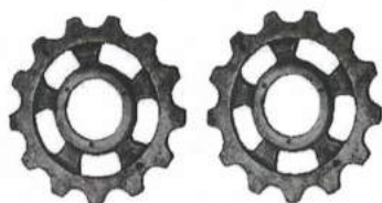
Звёздочка цепи для с/х цепных конвейеров ОСТ 32.194-2002
